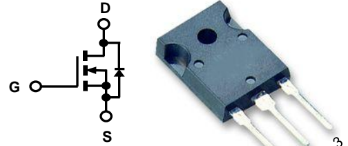
TO247 1:G, 2:D, 3:S, 4:D, (TO-247)
